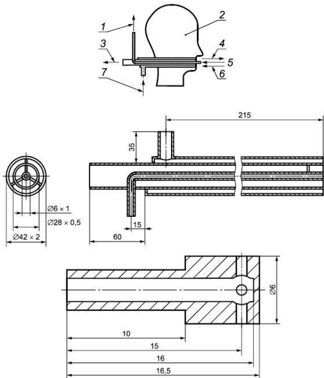
Рисунок 5 - Шеффилдский голова-манекен, предназначенный для определения содержания диоксида углерода во вдыхаемом воздухе, с трубкой для измерения сопротивления дыханию
