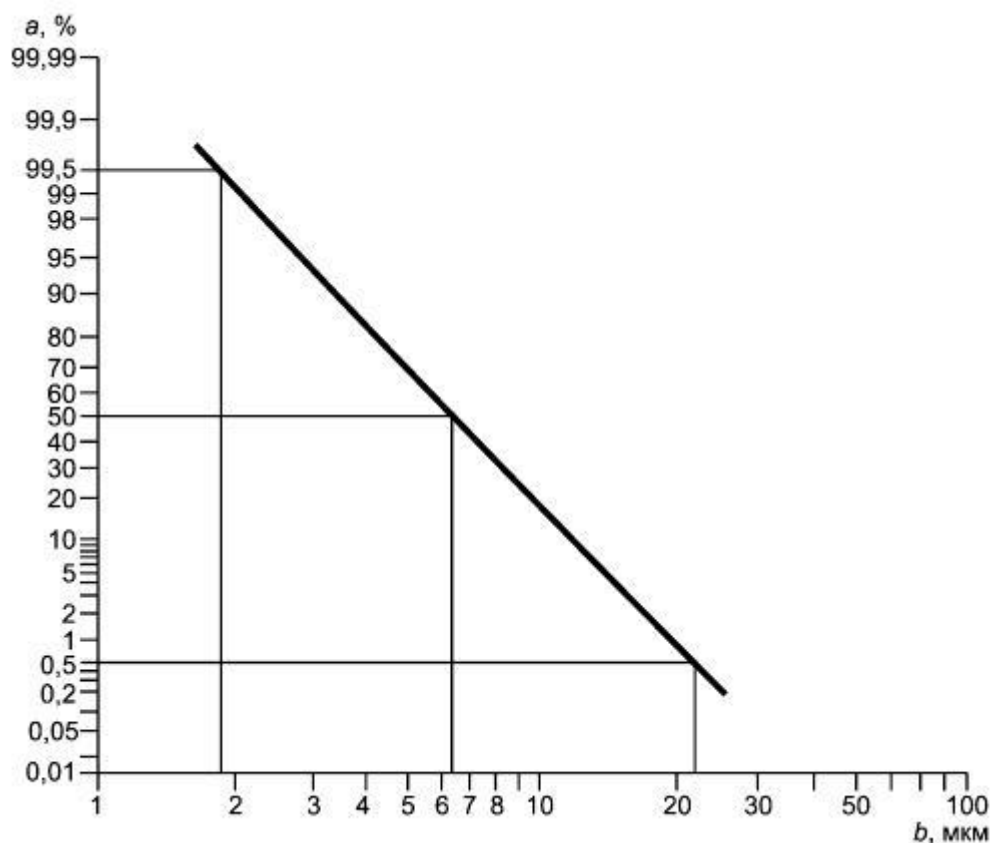
Рисунок 10 - Распределение частиц доломитовой пыли по размерам
