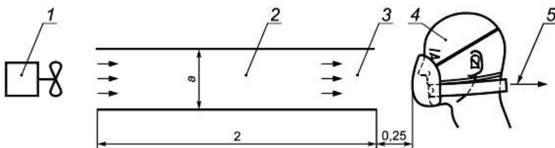
Рисунок 7 - Схема проведения испытания по определению содержания диоксида углерода
