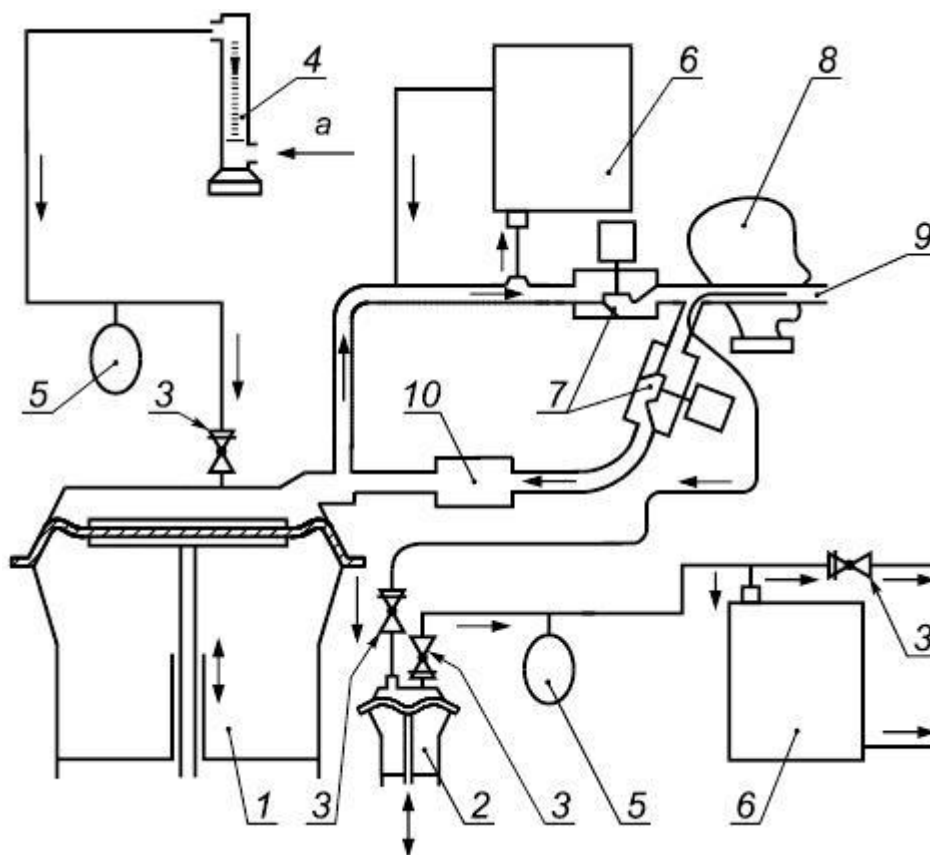
Рисунок 6 - Типовая схема испытательной установки для определения содержания диоксида углерода
